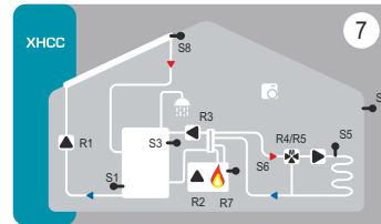
7 DHK Isıtma devresi, 3 yollu Vana ve Kazan ve Pompasının Kontrolü - Dağıtım Kolektörü ile Kullanım Sıcak Suyu Hazırlama ilave Solar Sistem Kontrolü
