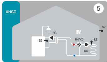
5 DHK Isıtma devresi, 3 yollu Vana Kontrol. Dağıtım Kolektörü ile Kullanım Sıcak Suyu Hazırlama
