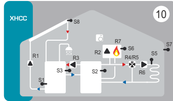
10 DHK Isıtma devresi, Kazan ve 3 yollu Vana Kontrolü Buffer Tank Uygulaması Solar Çift Serpantinli Boyler ile Kullanım Sıcak Suyu Hazırlama
