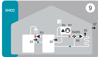
9 DHK Buffer Tank Isıtma devresi, 3 Yollu Vana Isı Pompası Kont. - Boylerli Kull. Sıcak Su Haz.
