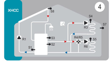
4 DHK Kombine Boylerli 2 Isıtma devresi, 3 Yollu Vana Kont. - Solar Sıcak Su Hazırlama Sistem Kontrolü
