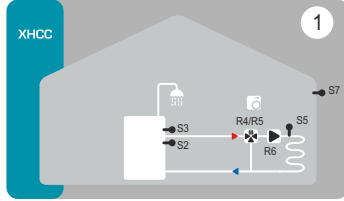
1 DHK Kombine Boylerli Isıtma devresi, 3 Yollu Vana Kont. - Kull. Sıcak Su Hazırlama Sistemi
