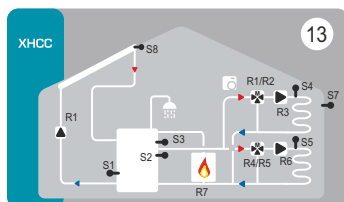
13 DHK 2 Zon Isıtma devresi, Kazan ve 3 yollu Vana Kontrolü (Farklı iki Sıcaklık devresi) Solar Kombine Boyler Kullanım Sıcak Suyu Hazırlama
