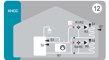
12 DHK 2 Zon Isıtma devresi, İki 3 yollu Vana Kontrolü - Kombine Boylerli - Isı Pompalı Kullanım Sıcak Suyu Hazırlama
