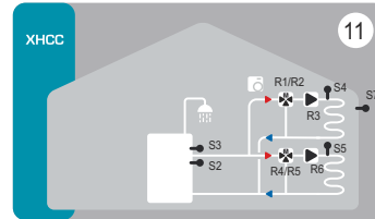
11 DHK 2 Zon Isıtma devresi, İki 3 yollu Vana Kontrolü - Kombine Boylerli Kullanım Sıcak Suyu Hazırlama
