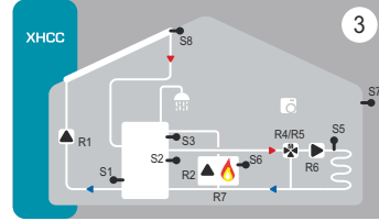
3 DHK Kombine Boylerli Isıtma devresi, 3 Yollu Vana, Kazan ve Pompası Kont. ilave Solar Sıcak Su Hazırlama Sistem Kontrolü
