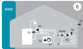
6 DHK Isıtma devresi, 3 yollu Vana ve Isı Pompası Kontrolü Dağıtım Kolektörü ile Kullanım Sıcak Suyu Hazırlama
