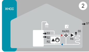
2 DHK Kombine Boylerli Isıtma devresi, 3 Yollu Vana ve Isı Pompası Kont. - Kull. Sıcak Su Hazırlama Sistemi
