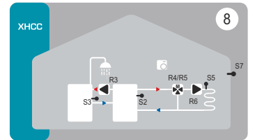
8 DHK Buffer Tank Isıtma devresi, 3 Yollu Vana Kont. - Boylerli Kull. Sıcak Su Hazırlama
